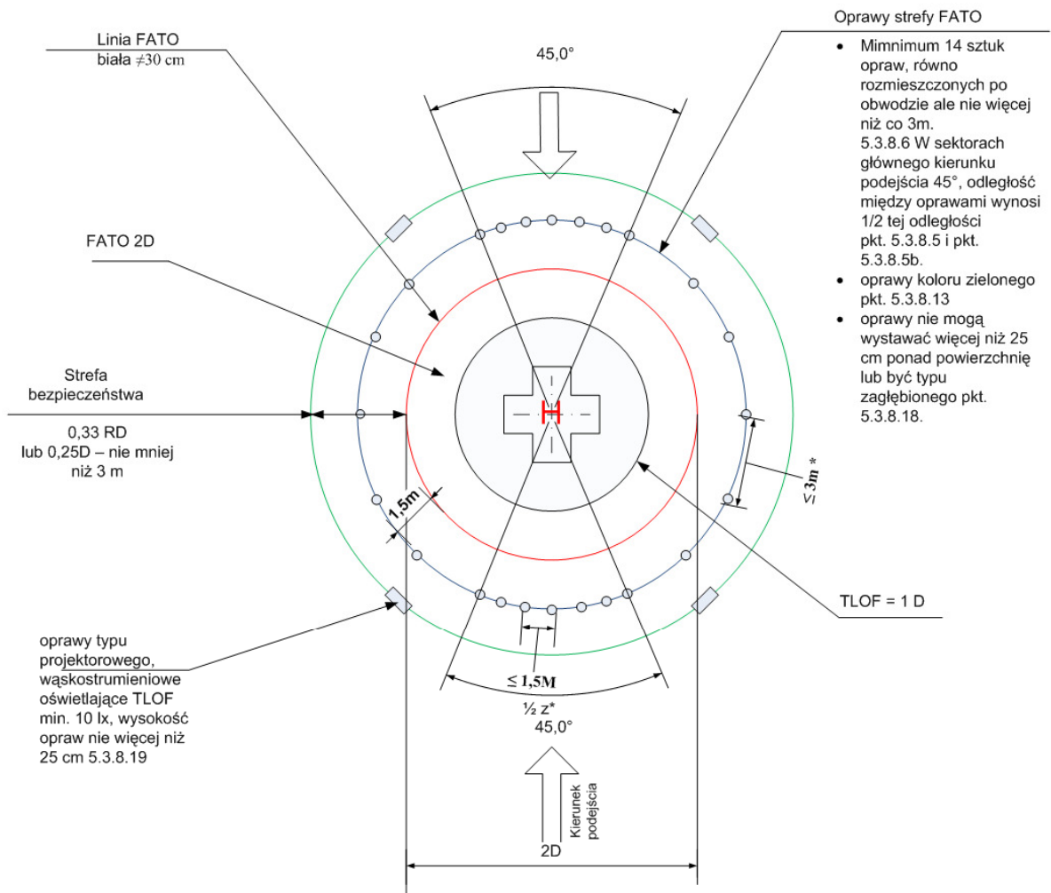
Rys Nr przykładowy widok ładowiska wyniesionego w formie okręgu
